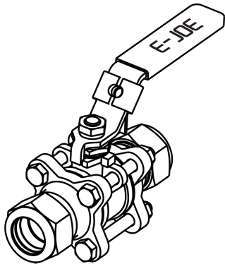
05、07、11、13、15、20 口径带锁定装置的球阀示意图
