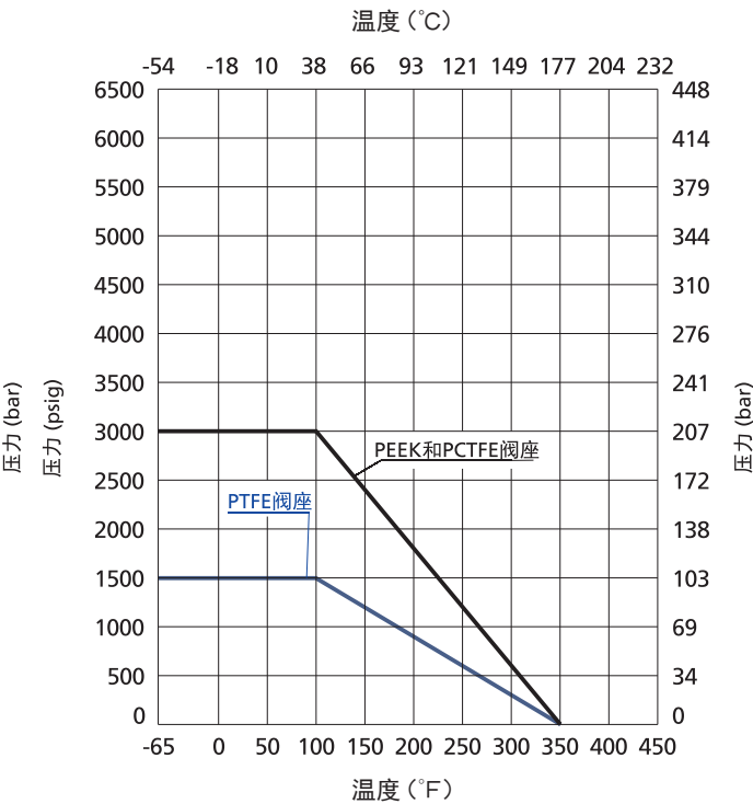
黄铜阀体
