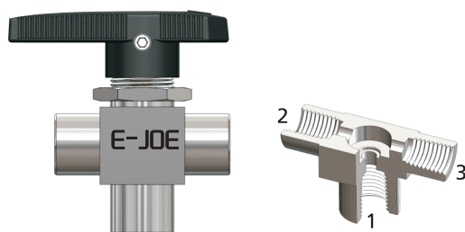
3 通阀门
