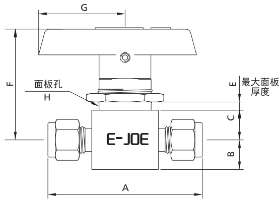
直通型
