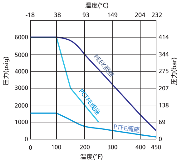
316 不锈钢阀体
