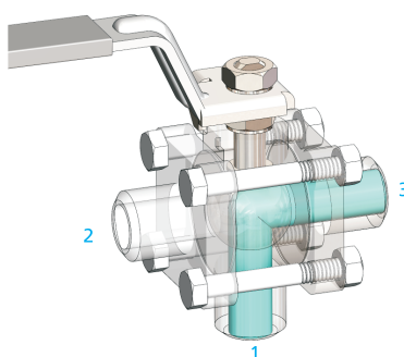
端口 1 和 3 连通
