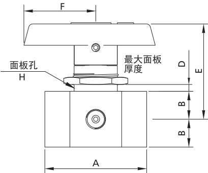
4 通阀门
