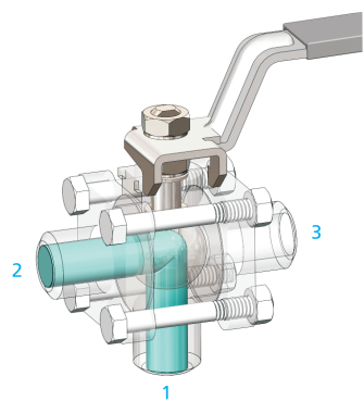
端口 1 和 2 连通
