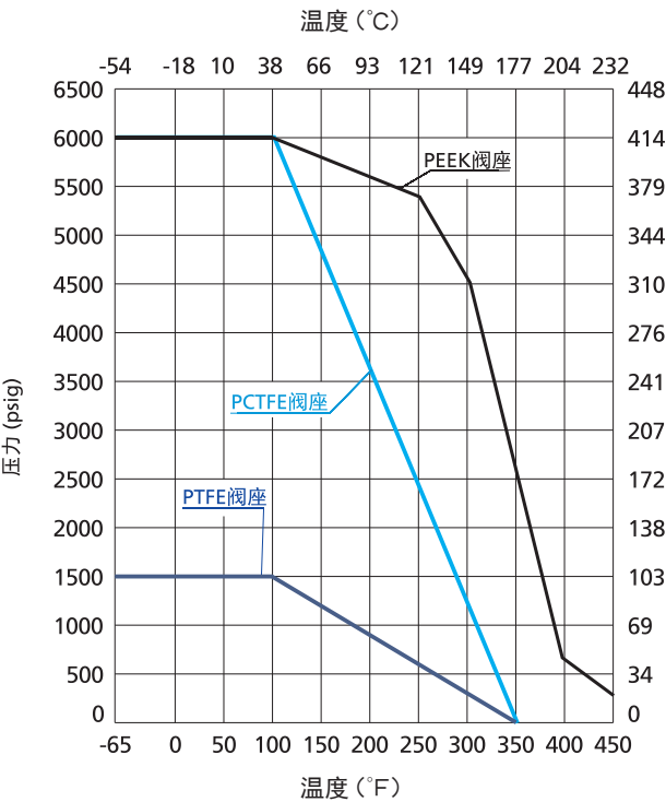
316 不锈钢阀体
