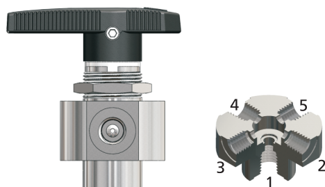
5 通阀门
