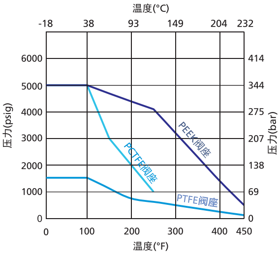
合金 400 阀体
