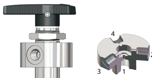
4 通阀门
