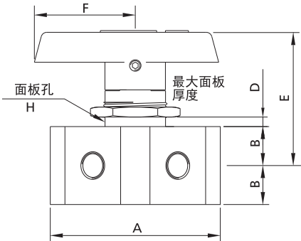
6 通阀门
