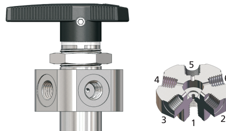
6 通阀门
