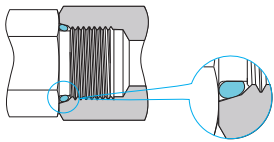
MST 阳螺纹端和 ISO 6149-1 端口
