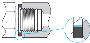
BS 阳螺纹端, BS 垫片和 BR 端口
