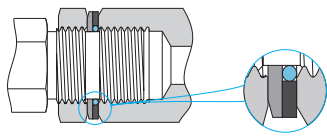
PP 阳螺纹端和 BR 端口
