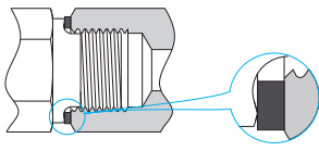
BR 阳螺纹端, BR 垫片和 BR 端口
