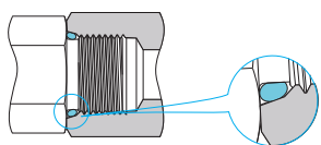
ST/SH 阳螺纹端和 SAE J1926-1 端口
