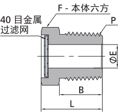
◆ 40 目 300 系列不锈钢过滤网组件
