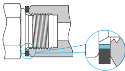
MRS 阳螺纹端, BS-M 垫片和 MS 端口
